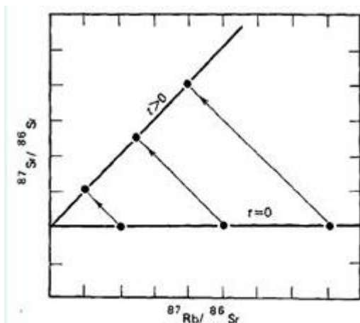
Рис. 8.1. Rb-Sr изохронная диаграмма, показывающая изотонную эволюцию пород во времени после их кристаллизации из однородной магмы.
